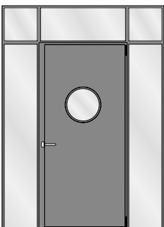
Verblechte einflügelige Türe mit festem Seitenteil und festen Oberlichtern Porte tôlée à un vantail avec avec partie latérale fixe et impostes fixes Sheet metal single leaf door with fixed side light and fixed top lights
