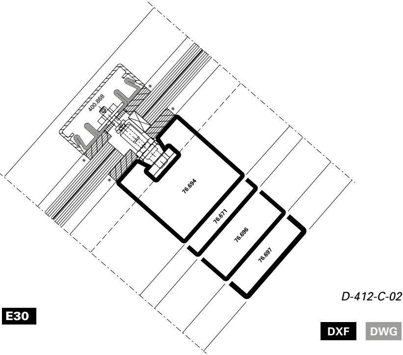
Riegel-Detail
