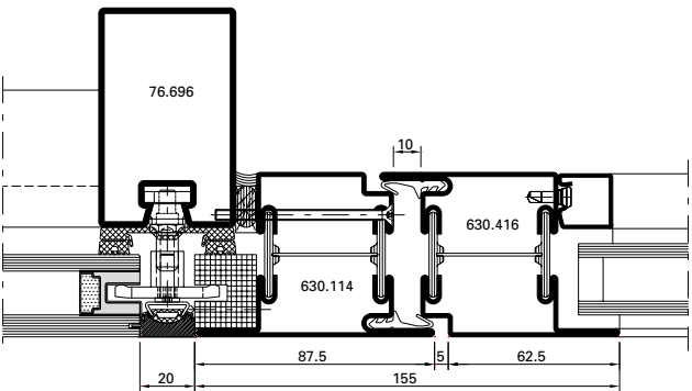
Einsatzelement Türe Elément de remplissage porte Infill element door
