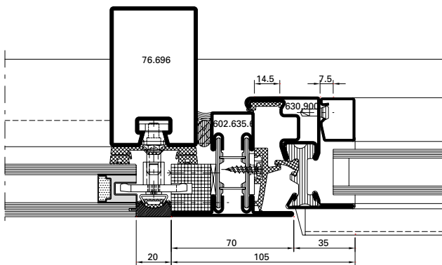
Einsatzelement Fenster Elément de remplissage fenêtre Infill element window
