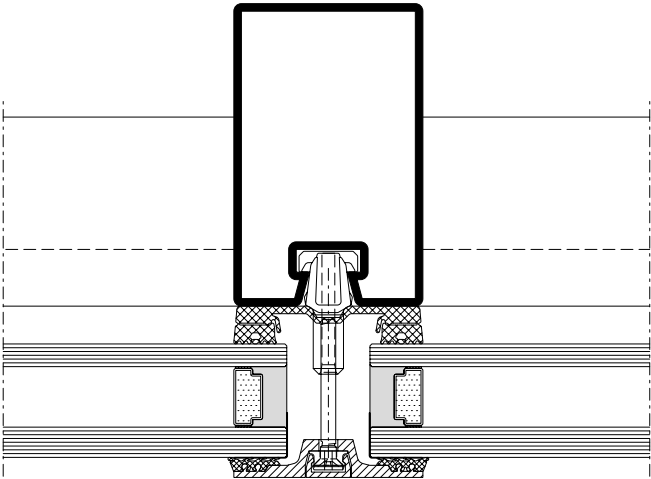
DXF DWG D-533-C-017
