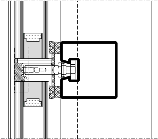
DXF DWG D-533-C-019
