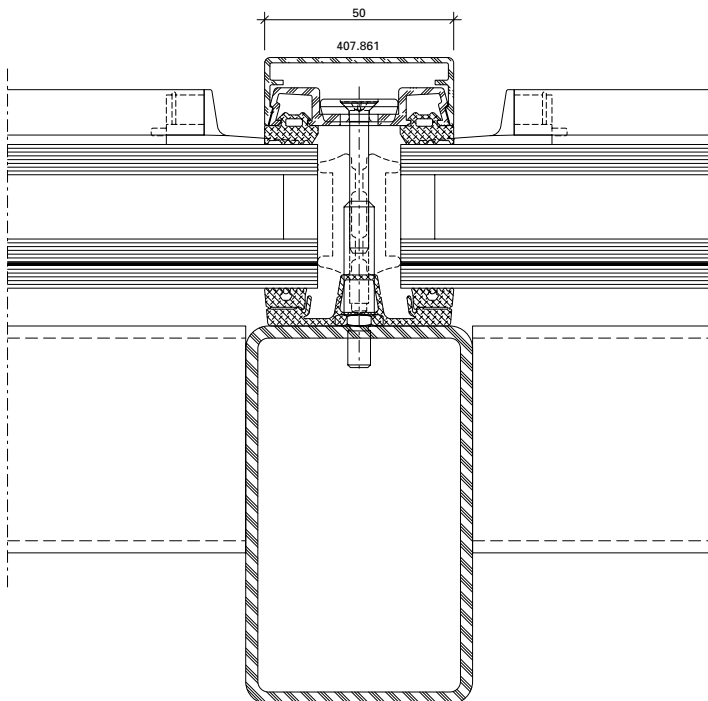
Détail du chevron Largeur de face 50 mm Goujon à visser
