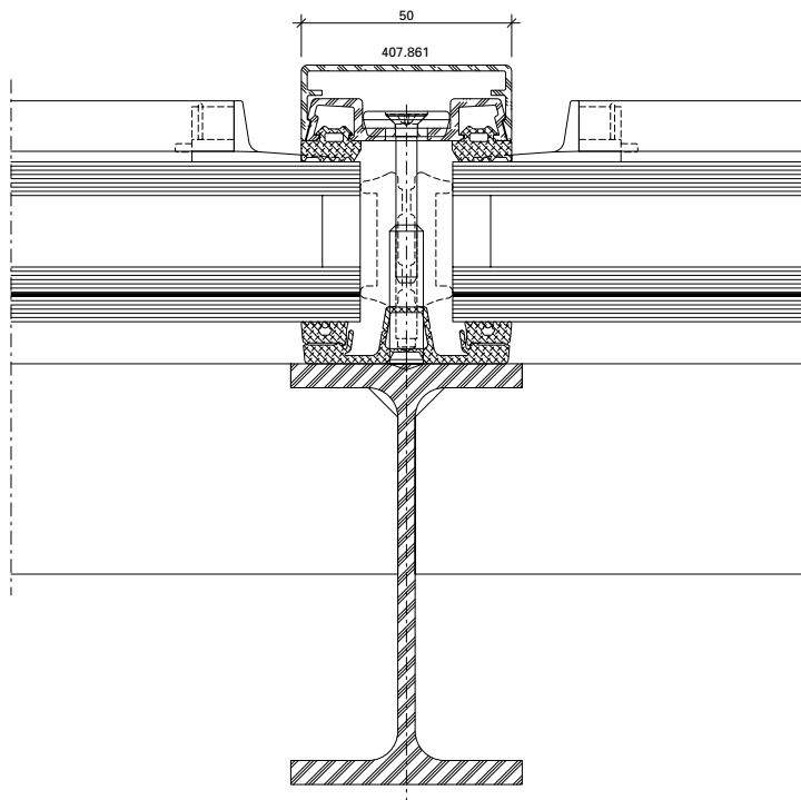
Riegel-Detail Ansichtsbreite 50 mm Schweissbolzen
