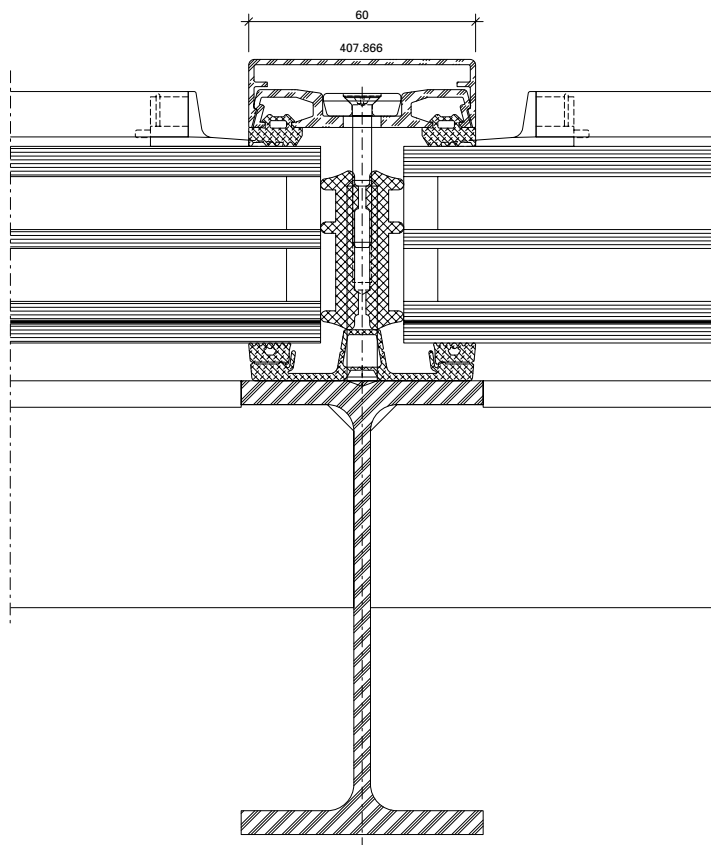
Détail du chevron HI Largeur de face 60 mm Goujon à souder
