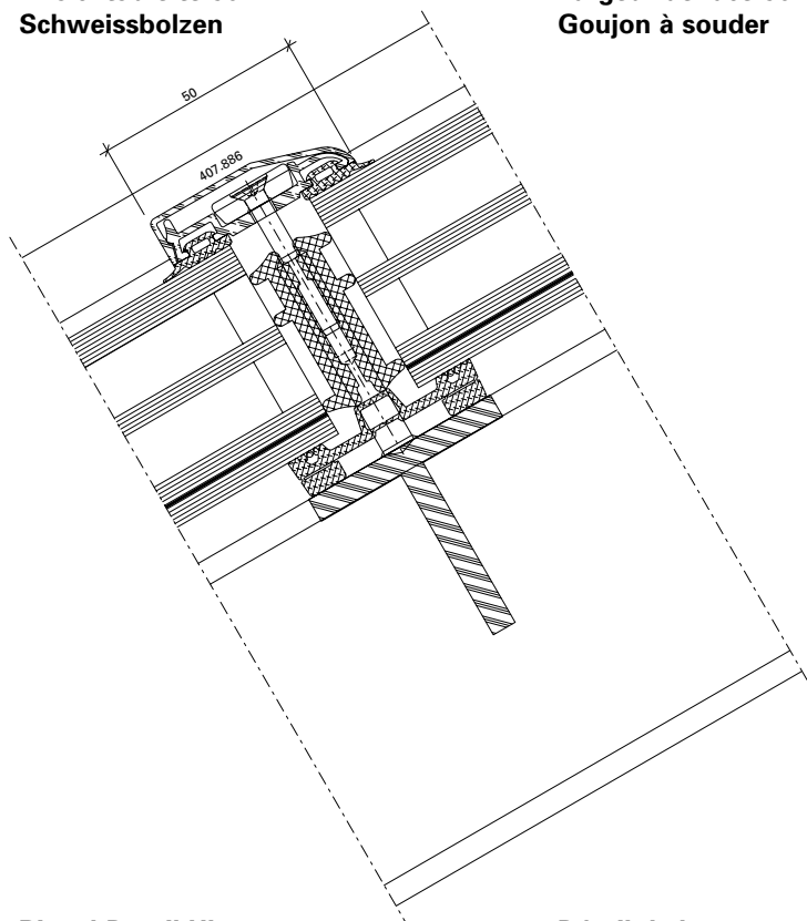
Riegel-Detail HI Ansichtsbreite 50 mm Schweissbolzen
