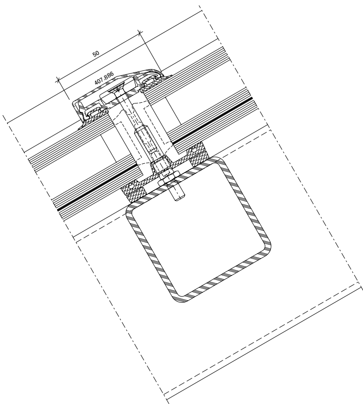
Détail de la traverse Largeur de face 50 mm Goujon à visser
