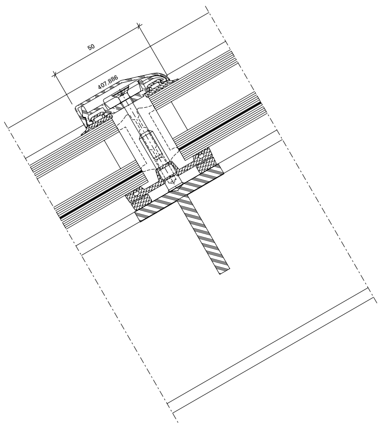
Détail de la traverse Largeur de face 50 mm Goujon à souder
