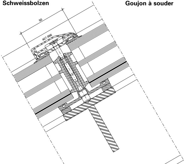
Riegel-Detail HI Ansichtsbreite 50 mm Schweissbolzen
