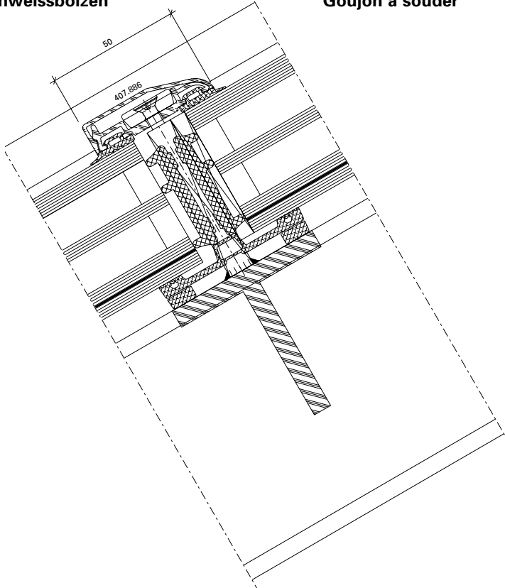
Riegel-Detail HI Ansichtsbreite 50 mm Schweissbolzen
